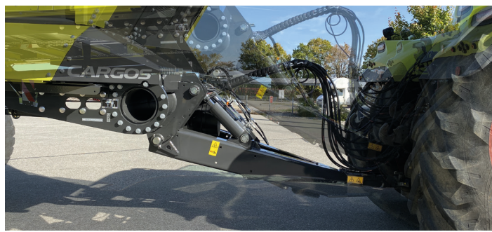
Timon articulé à la manière d'un essieu relevable Sytem-braquage
