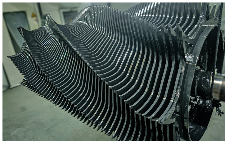
Neuf rangées de dents enfichées et fixées sur le manteau du rotor. dents de rotor vissées
