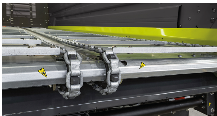
Chaînes de fond mouvant galvanisées, résistantes à la charge et à la déchirure
