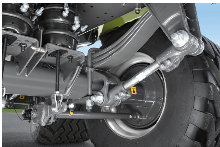
Version mécanique suspension à ressort.
